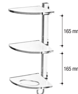
606 Angolare doccia Shower corner tray L. 160 H. 460 P. 172 mm
