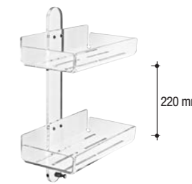
1222 - 1232 Portaoggetti Accessory holder 1222 - L. 210 H. 430 P. 155 mm 1232 - L. 310 H. 430 P. 155 mm
