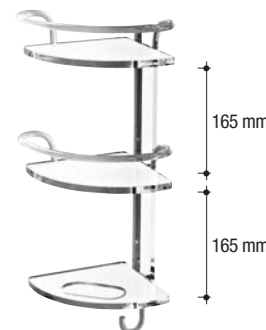
604 Angolare doccia Shower corner tray L. 160 H. 485 P. 172 mm
