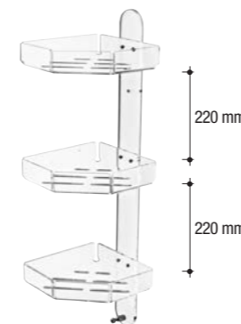
1213 Angolare doccia Shower corner tray L. 185 H. 630 P. 195 mm
