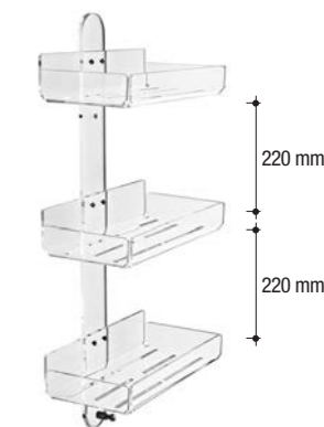
1223 - 1233 Portaoggetti Accessory holder 1223 - L. 210 H. 630 P. 155 mm 1233 - L. 310 H. 630 P. 155 mm
